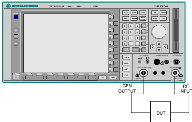
Bild 4-25 Anordnung für Transmissionsmessungen
