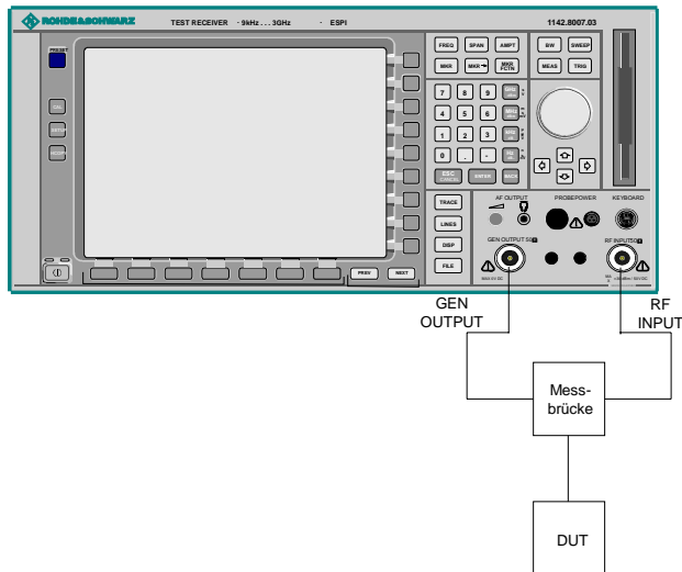
Bild 4-31 Anordnung für Reflexionsmessungen
