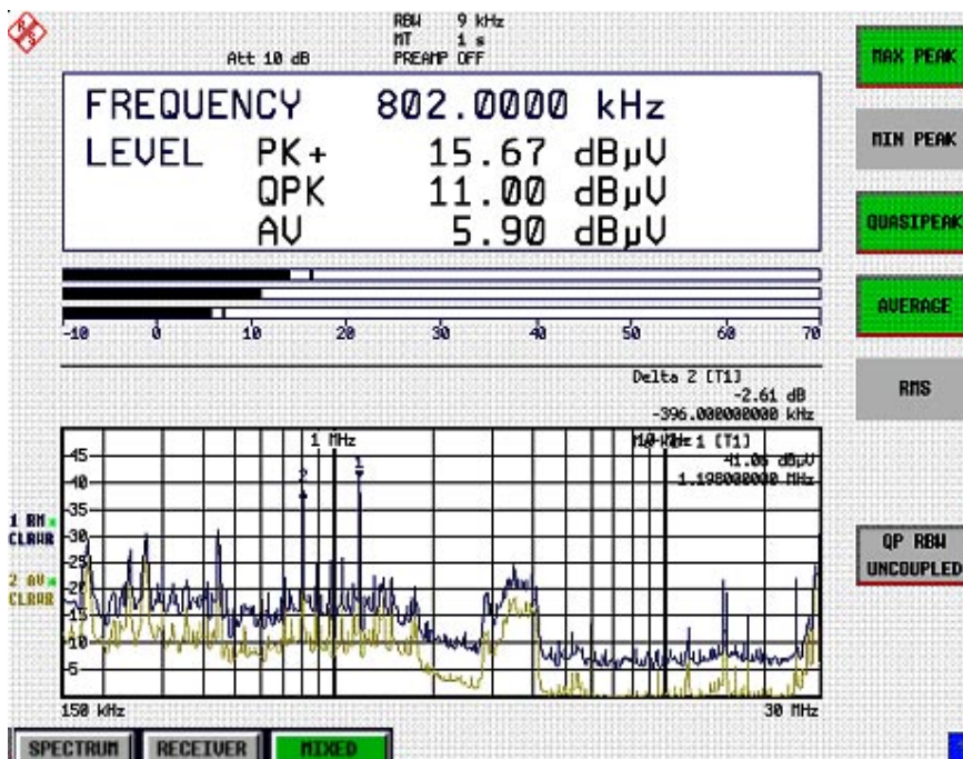
Bild 3-4 Bildschirmaufteilung des R&S ESCI in Split Screen-Darstellung
