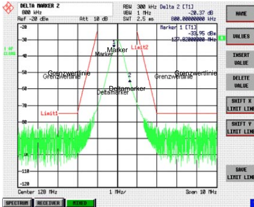
Bild 3-3 Messdiagramm
