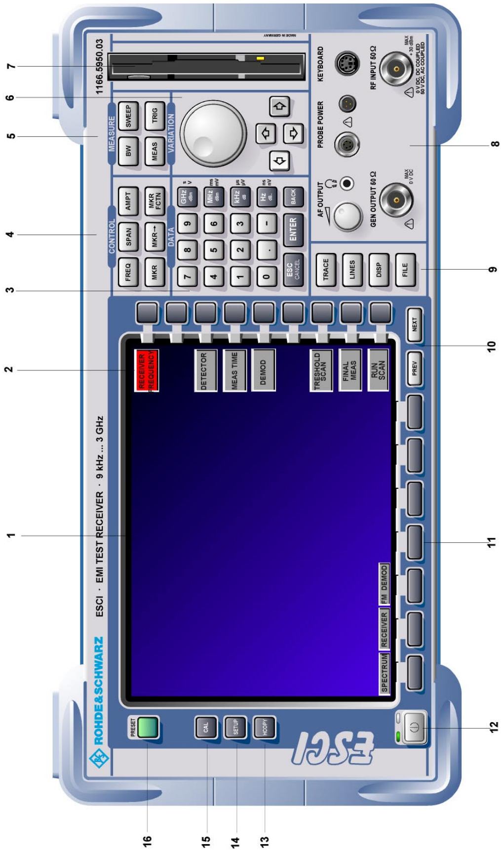
Bild 1-1 Frontansicht
