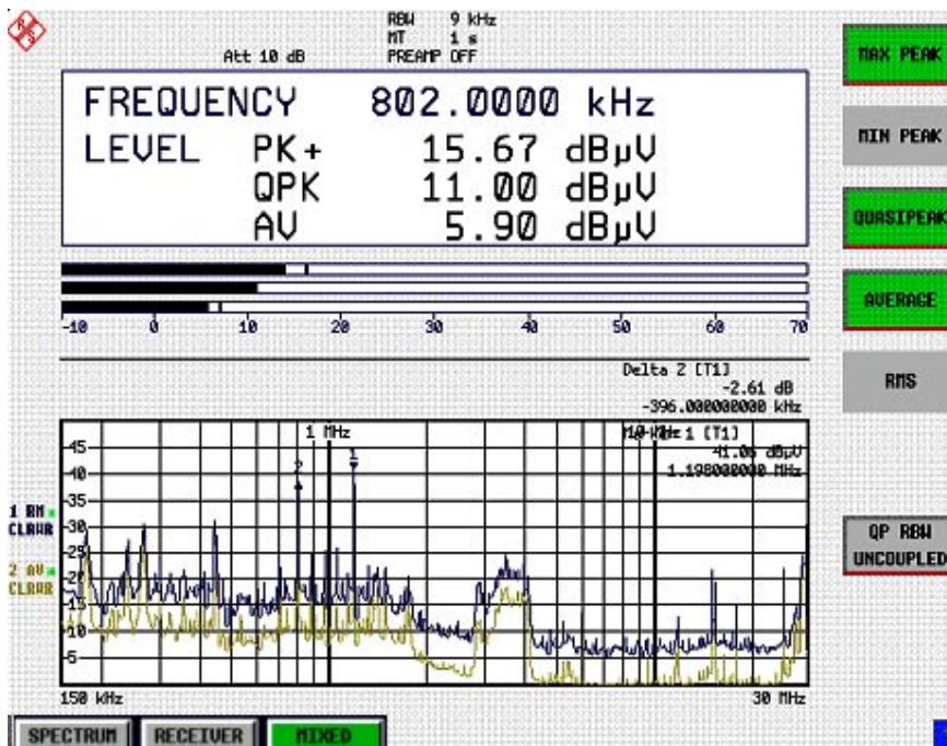
Bild 4-21 Beispiel für eine Darstellung von 2 Messfenstern (Split Screen). Die Einstellungen sind nicht gekoppelt
