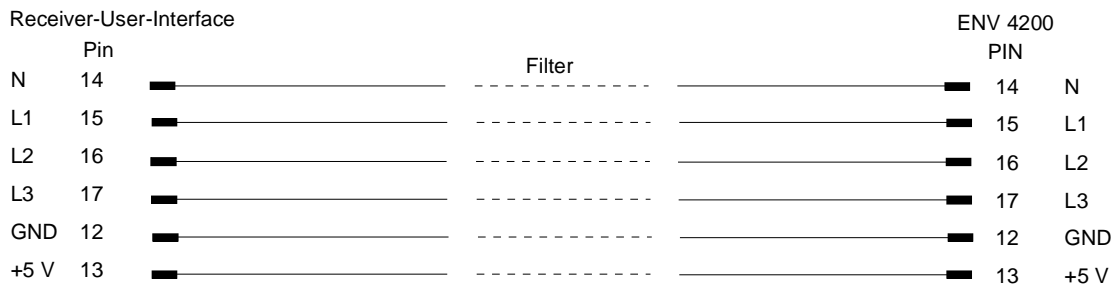
Bild 4-5 Verbindung R&S ESCI mit R&S ENV4200 (Zur Direktverbindung ohne Filter: Kabel R&S EZ-21)
