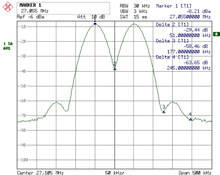
Bild 4-13 Beispiel für Pegelmessungen bei verschiedenen Einstellungen von Peak Excursion
