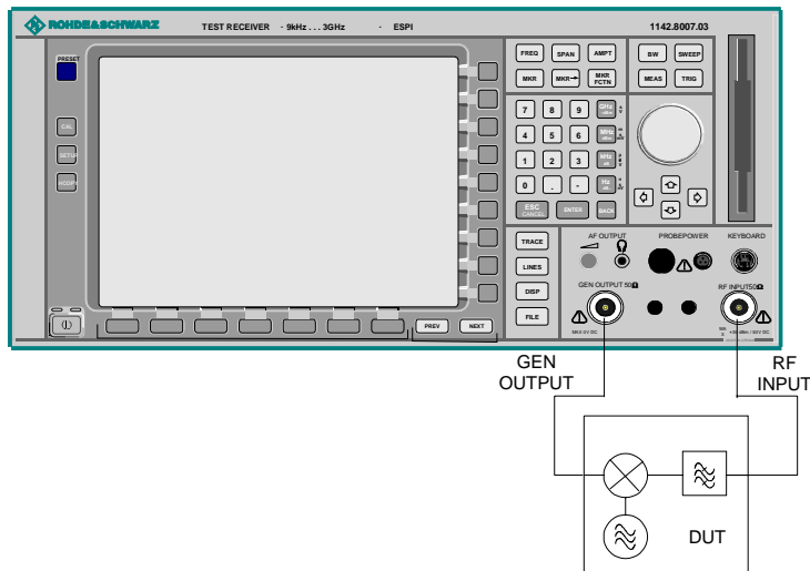
Bild 4-32 Anordnung für frequenzumsetzende Messungen
