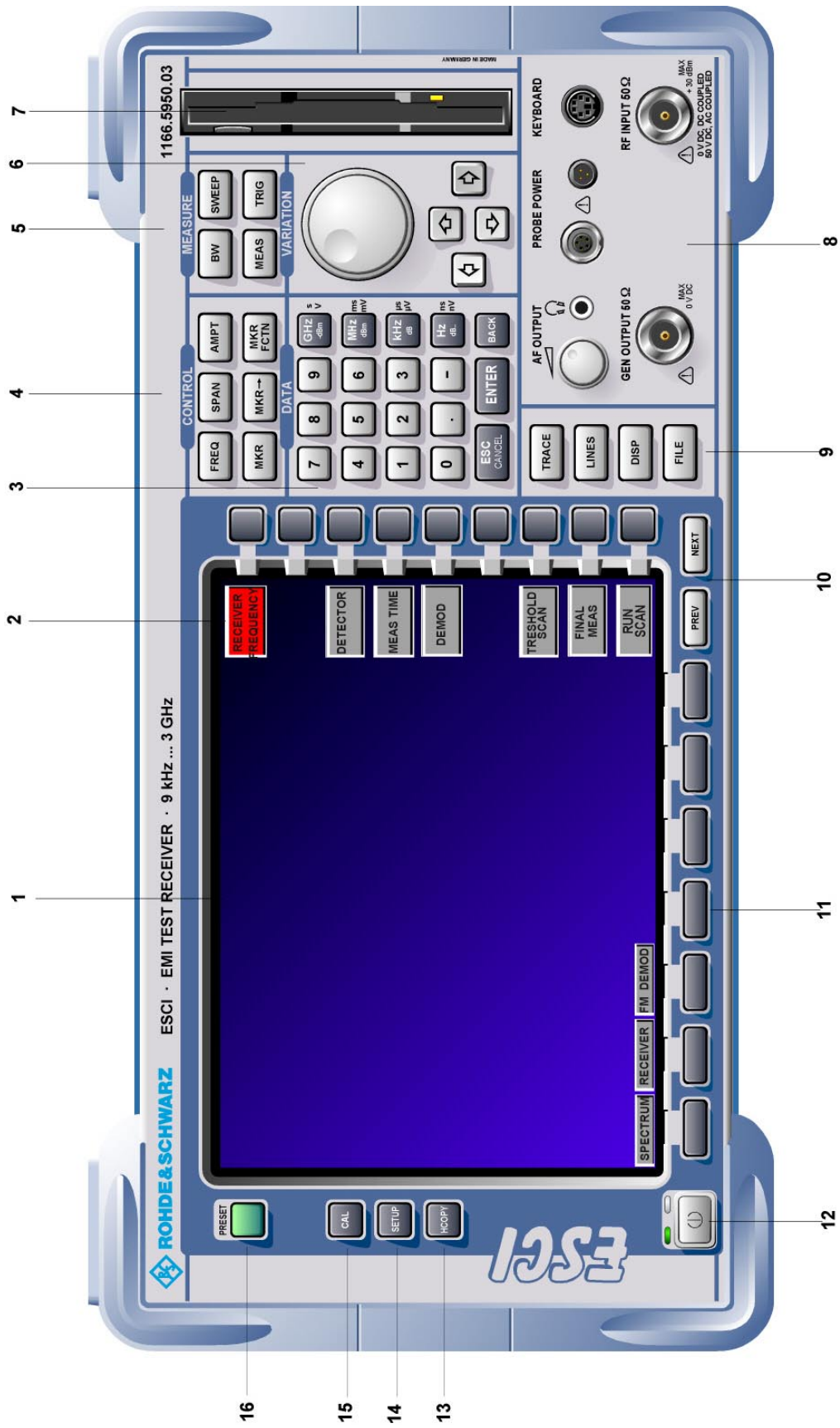
Bild 1-1 Frontansicht
