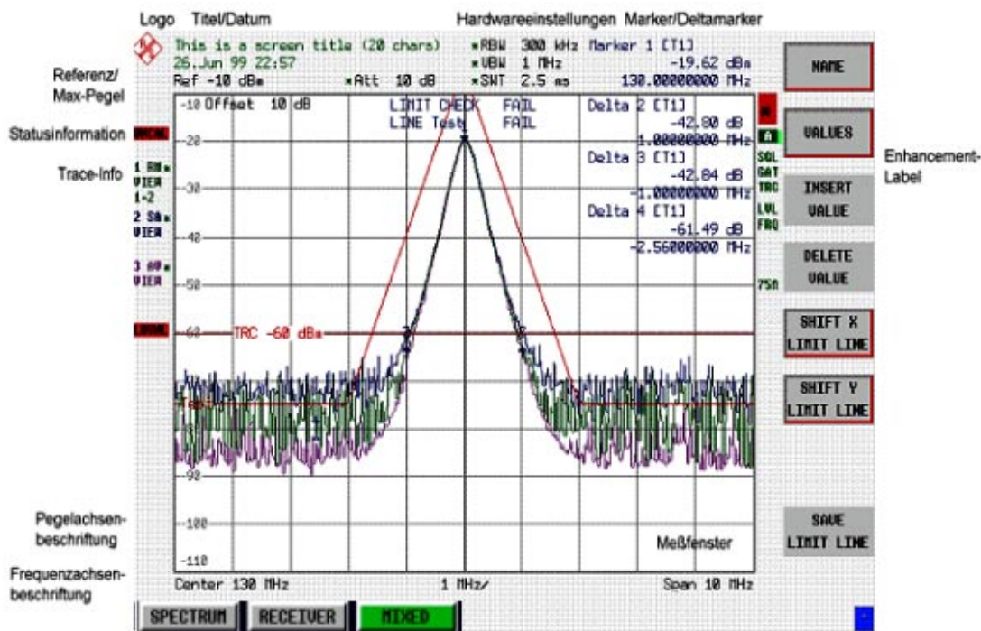
Bild 3-2 Bildschirmaufteilung des R&S ESCI im Analysatorbetrieb
