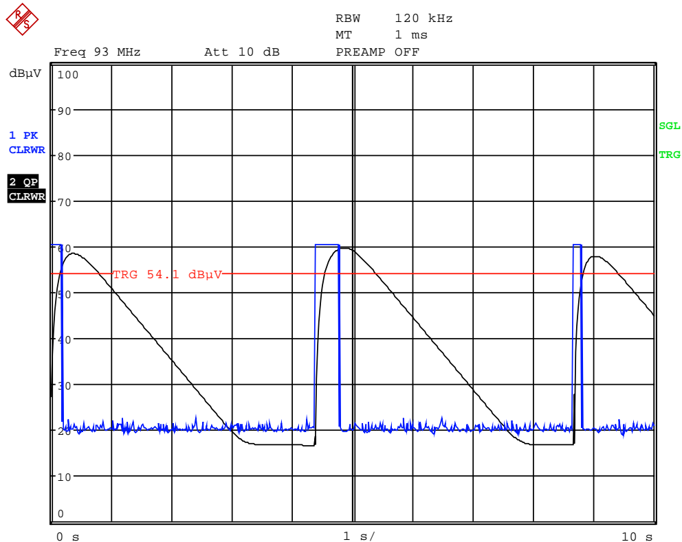
Bild 4-8 Scan im Zeitbereich
