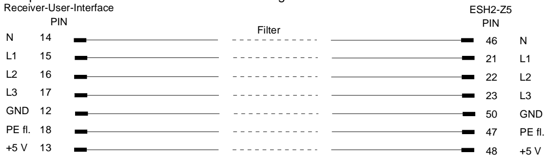
Bild 4-3 Verbindung R&S ESCI mit R&S ESH2-Z5 (zur Direktverbindung ohne Filter: Kabel R&S EZ-13)
