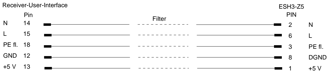
Bild 4-4 Verbindung R&S ESCI mit R&S ESH3-Z5 (Zur Direktverbindung ohne Filter: Kabel R&S EZ-14, Modell 02)
